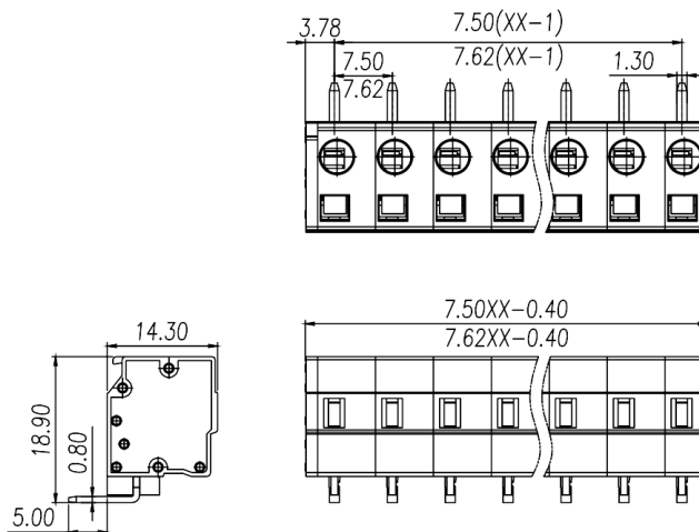
尺寸图 Dimensions
