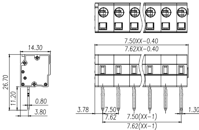
尺寸图 Dimensions
