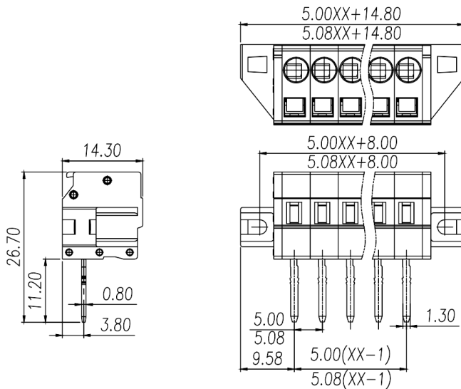
尺寸图 Dimensions
