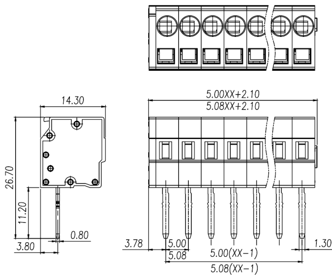
尺寸图 Dimensions
