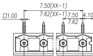
尺寸图 Dimensions
