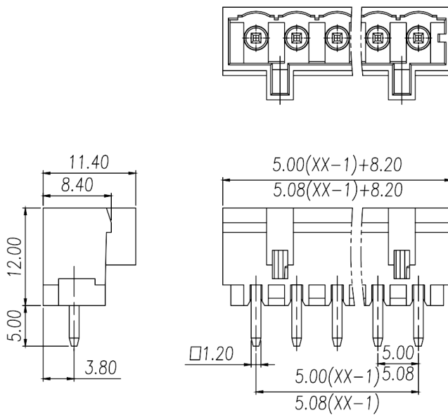
尺寸图 Dimensions
