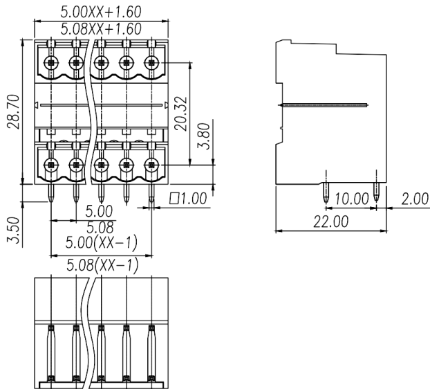
尺寸图 Dimensions
