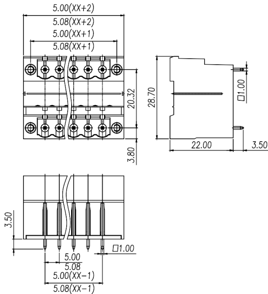
尺寸图 Dimensions
