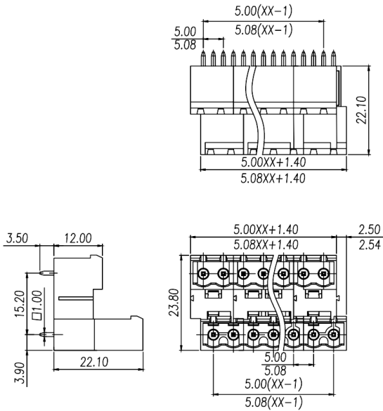
尺寸图 Dimensions
