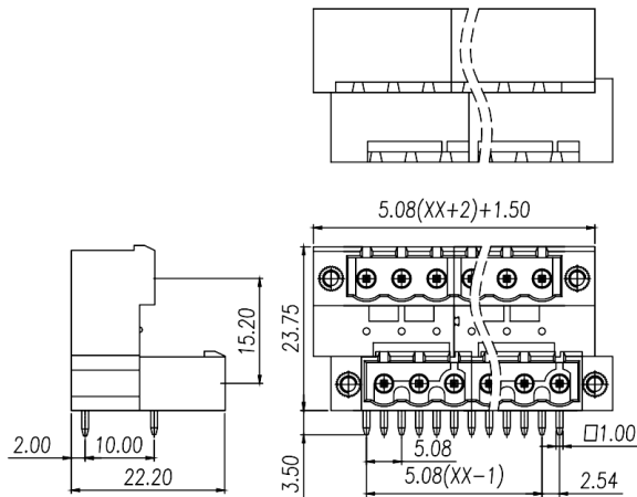
尺寸图 Dimensions
